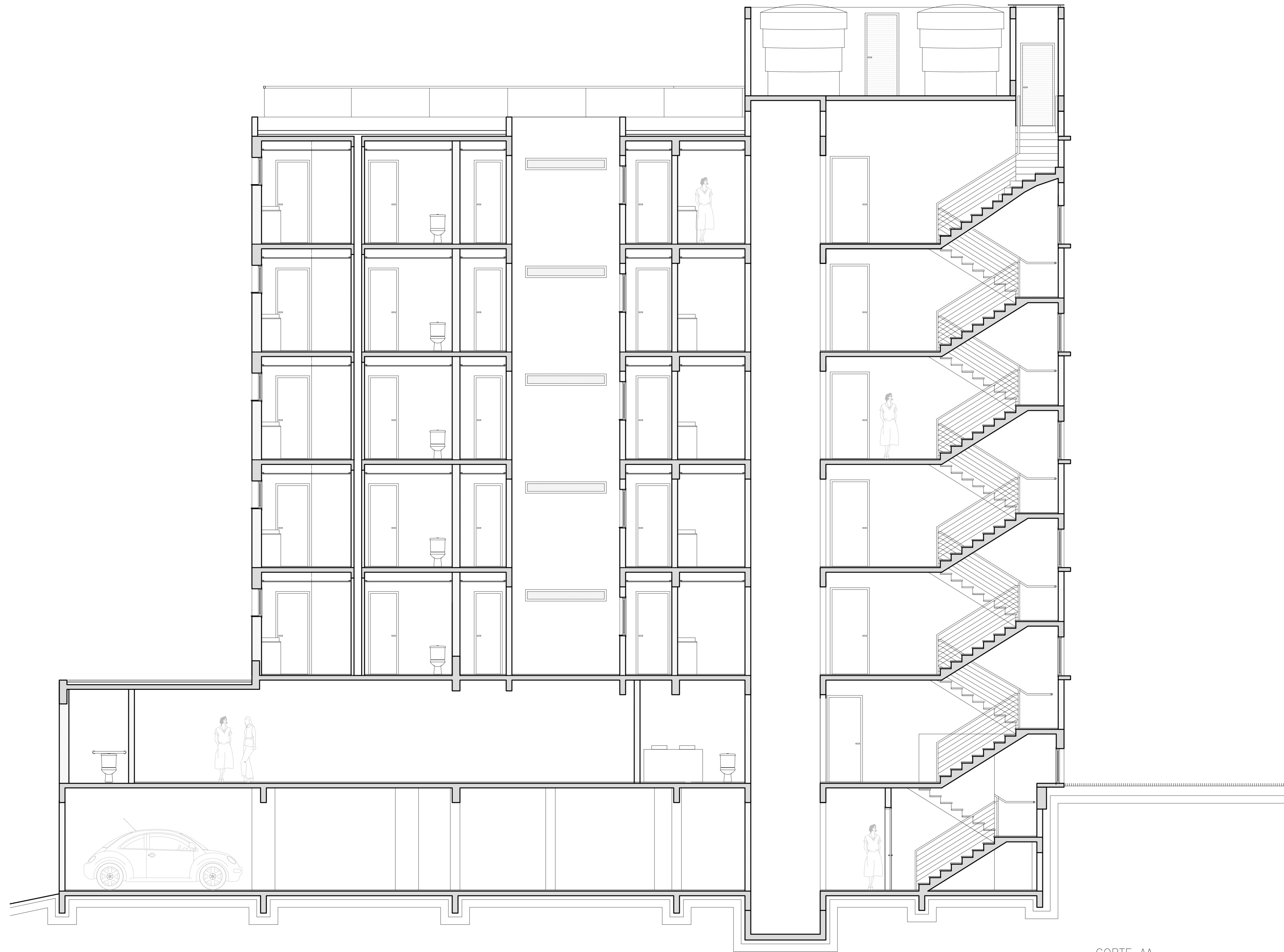
CORTE AA 0 1m 5m
