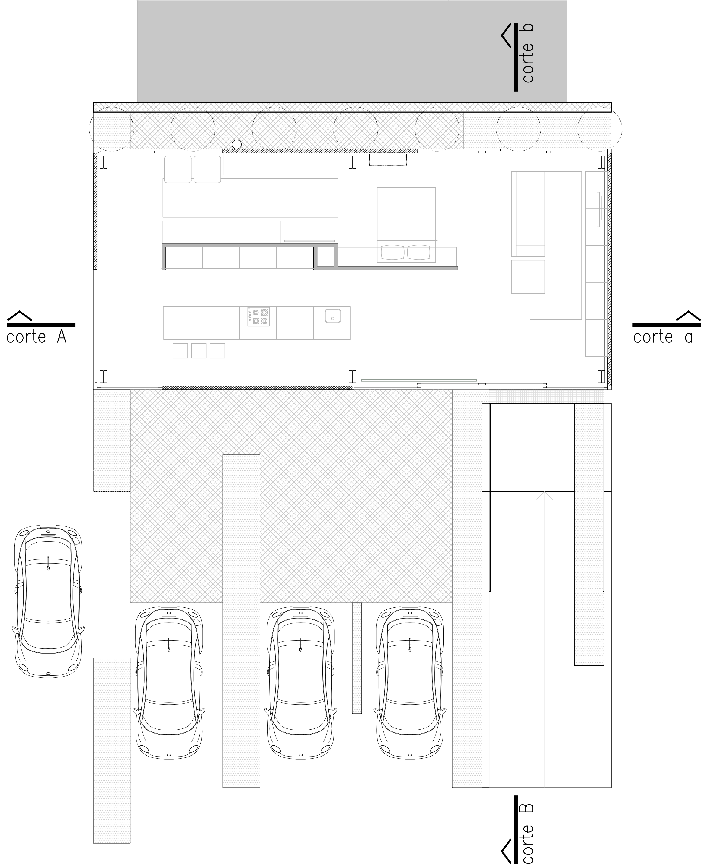
PLANTA BAIXA 0 1m 5m
