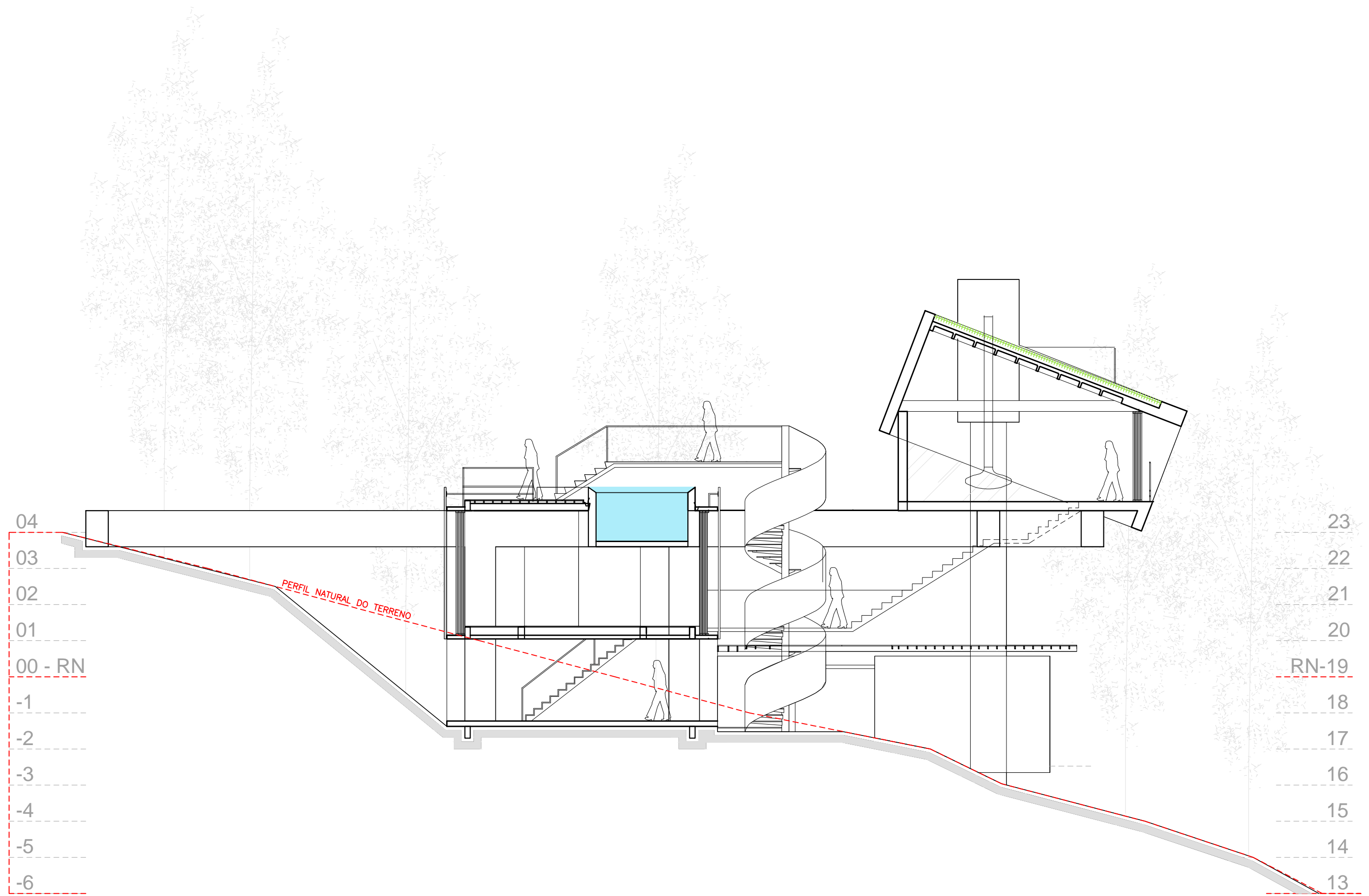
CORTE Aa 0 1m 5m
